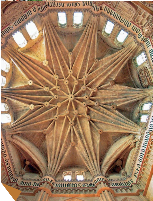
Bóveda estrellada de la Capilla de los Vélez
